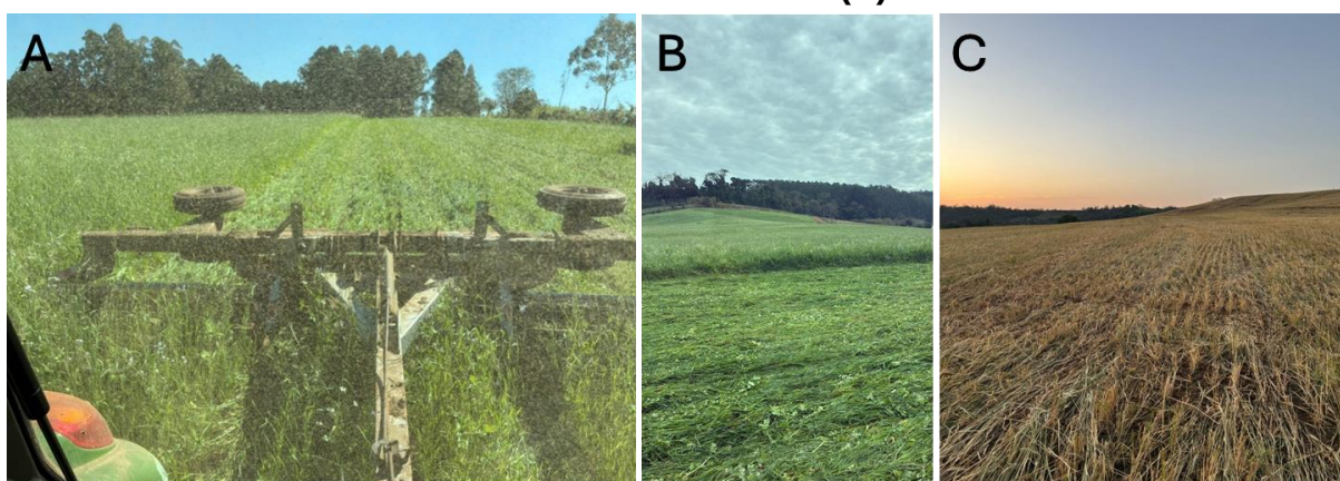
Figura 5 – Equipamento para rolagem das plantas de cobertura (A), plantas logo após o manejo (B) e condição da palhada no momento da semeadura (C).
