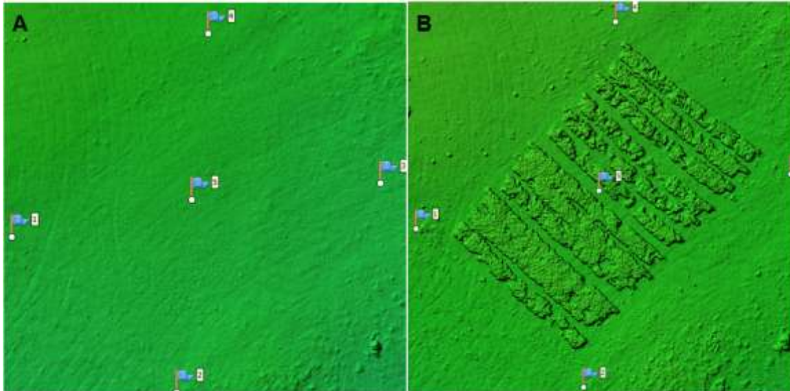
Figura 8- Comparativo dos modelos digitais de elevação.
